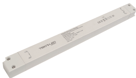
Ref : TL 24D 100 Alimentation 24Vdc ON/OFF DIM TRIAC Puissance max : 100W Dimensions : 330x30x23mm
