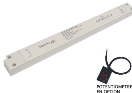
Ref : TL 24D 100 Alimentation 24Vdc ON/OFF DIM 0-1/10V Puissance max : 100W Dimensions : 330x30x23mm
