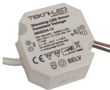
Ref : TL 24D 12 Alimentation 24Vdc ON/OFF DIM TRIAC Puissance max : 12W Dimensions : 60x50x25mm
