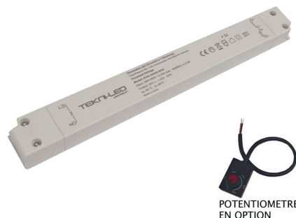
Ref : TL 24D 30 Alimentation 24Vdc ON/OFF DIM 0-1/10V Puissance max : 30W Dimensions : 260x30x20mm
