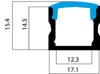
Ref : EVO2-OP / EVO2-TR Profilé haut
