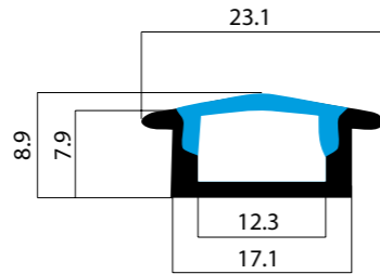
Ref : EVO-OP / EVO-TR Profilé encastrable
