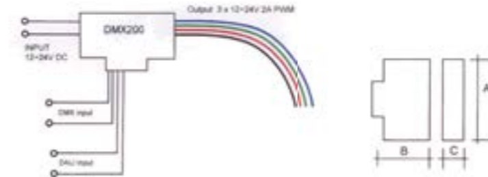
Ref : TL DMX 200
