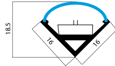
Ref : EVO3-OP Profilé d'angle
