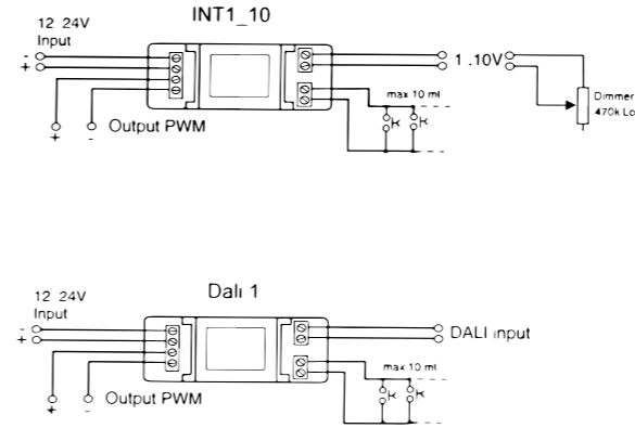
Ref : TL DC DALI / TL DC 1-10
